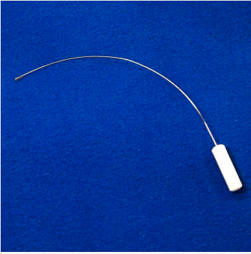
Einfädler für den Untergreifer
